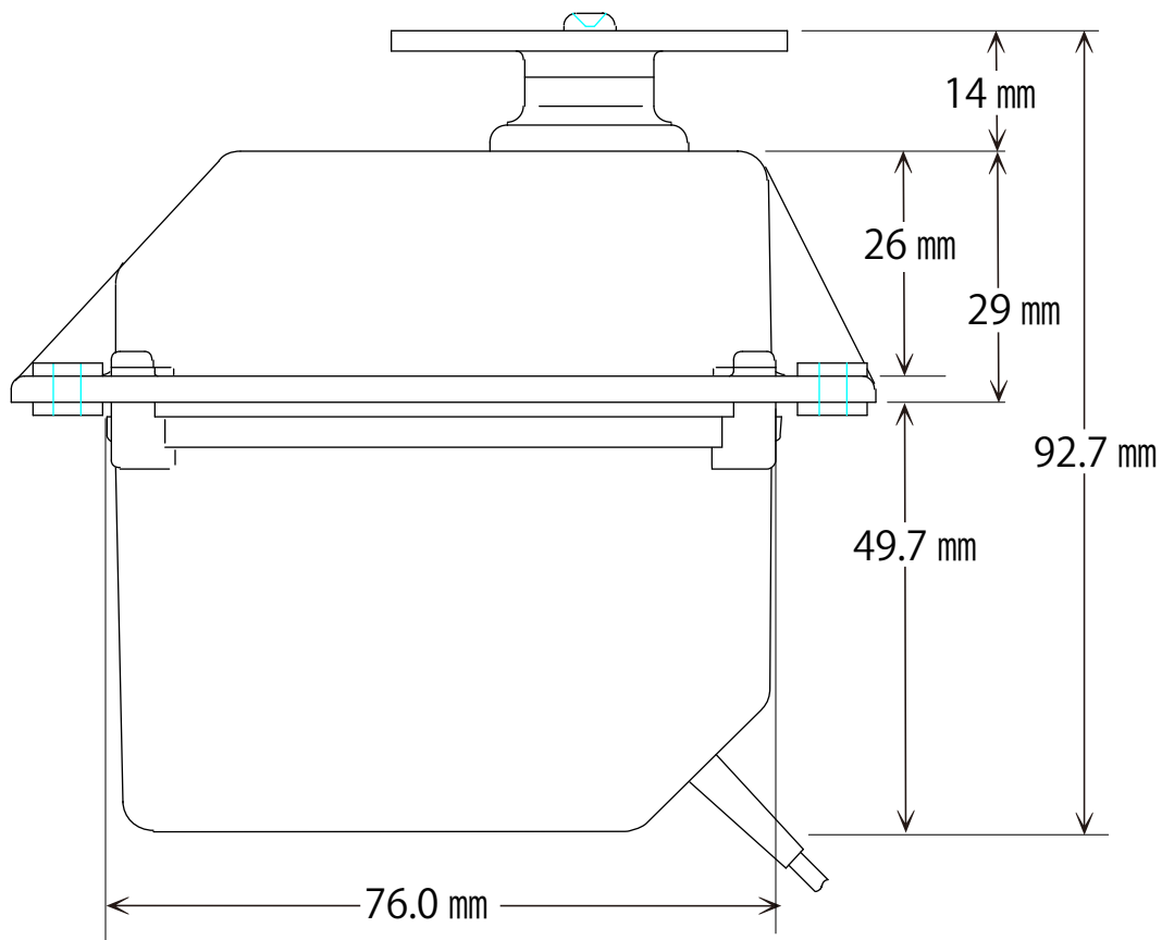
PS-050 寸法図
